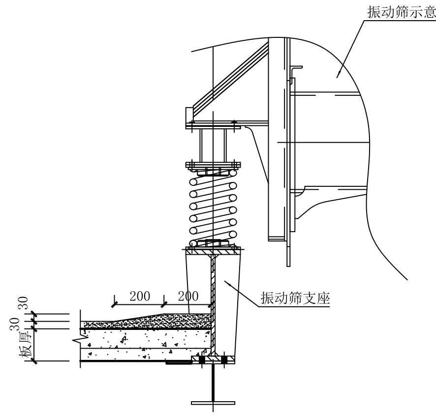
17 振动筛支座处楼板细部做法示意图
