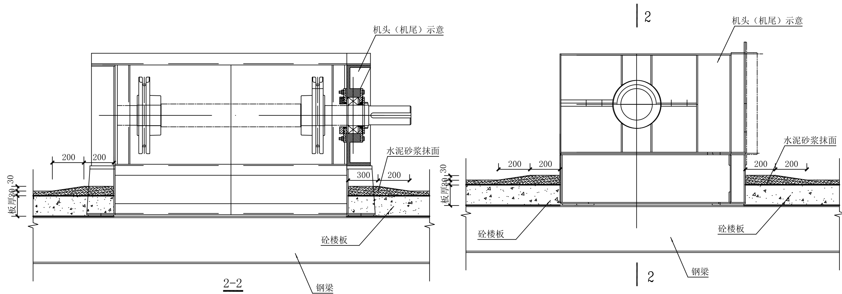
19 刮板、皮带机头机尾（支座式）处楼板细部做法示意图
