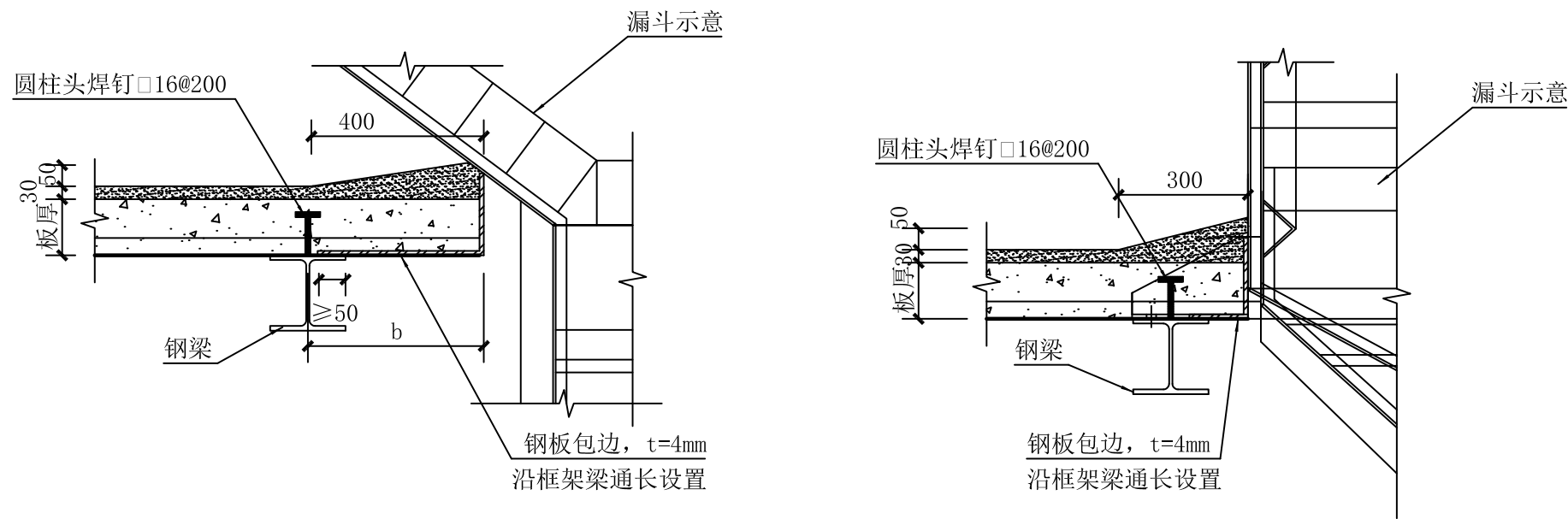
12 楼板端部与漏斗处楼板细部做法示意图
