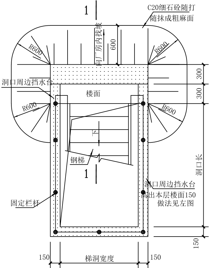
楼面钢梯洞口挡水台做法
