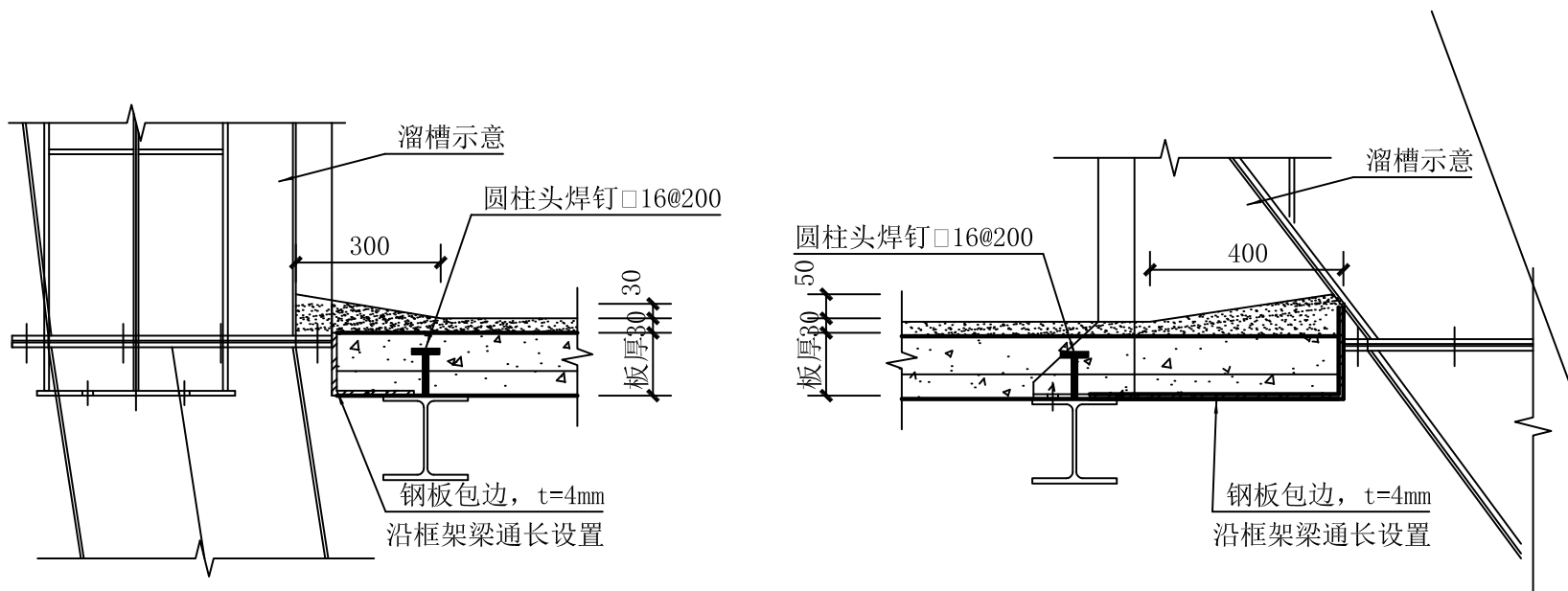
16 楼板端部与溜槽处楼板细部做法示意图
