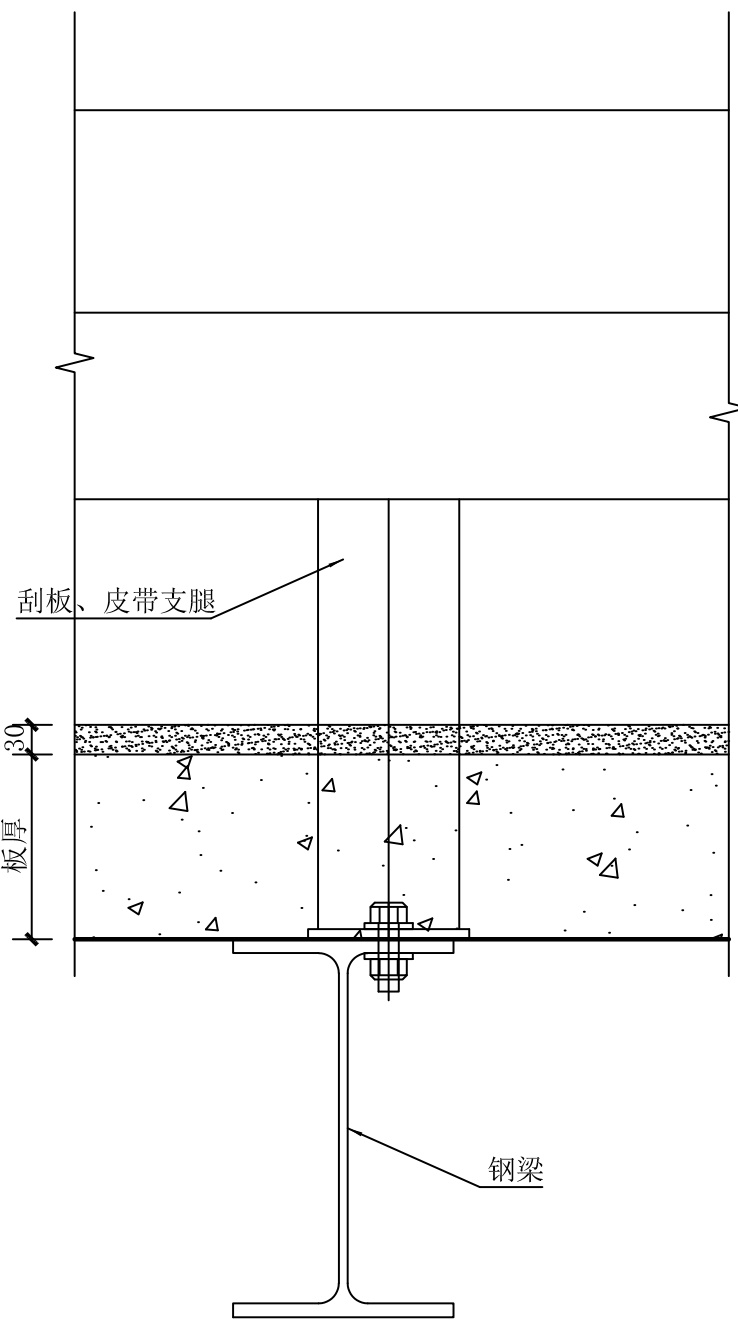
15 刮板、皮带支腿处楼板细部做法示意图
