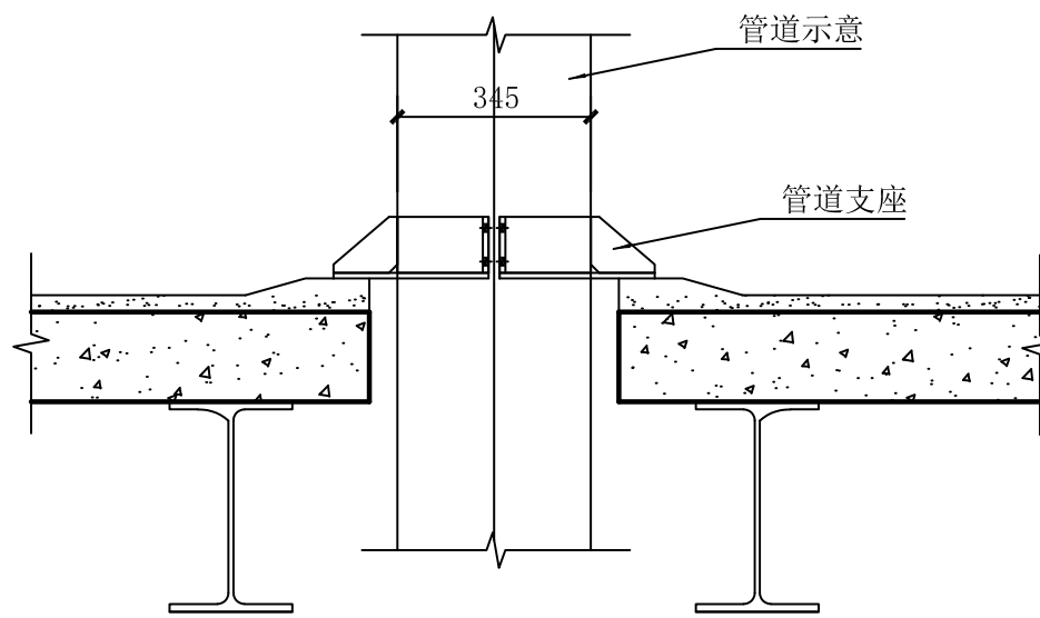
18 管道处楼板细部做法示意图
