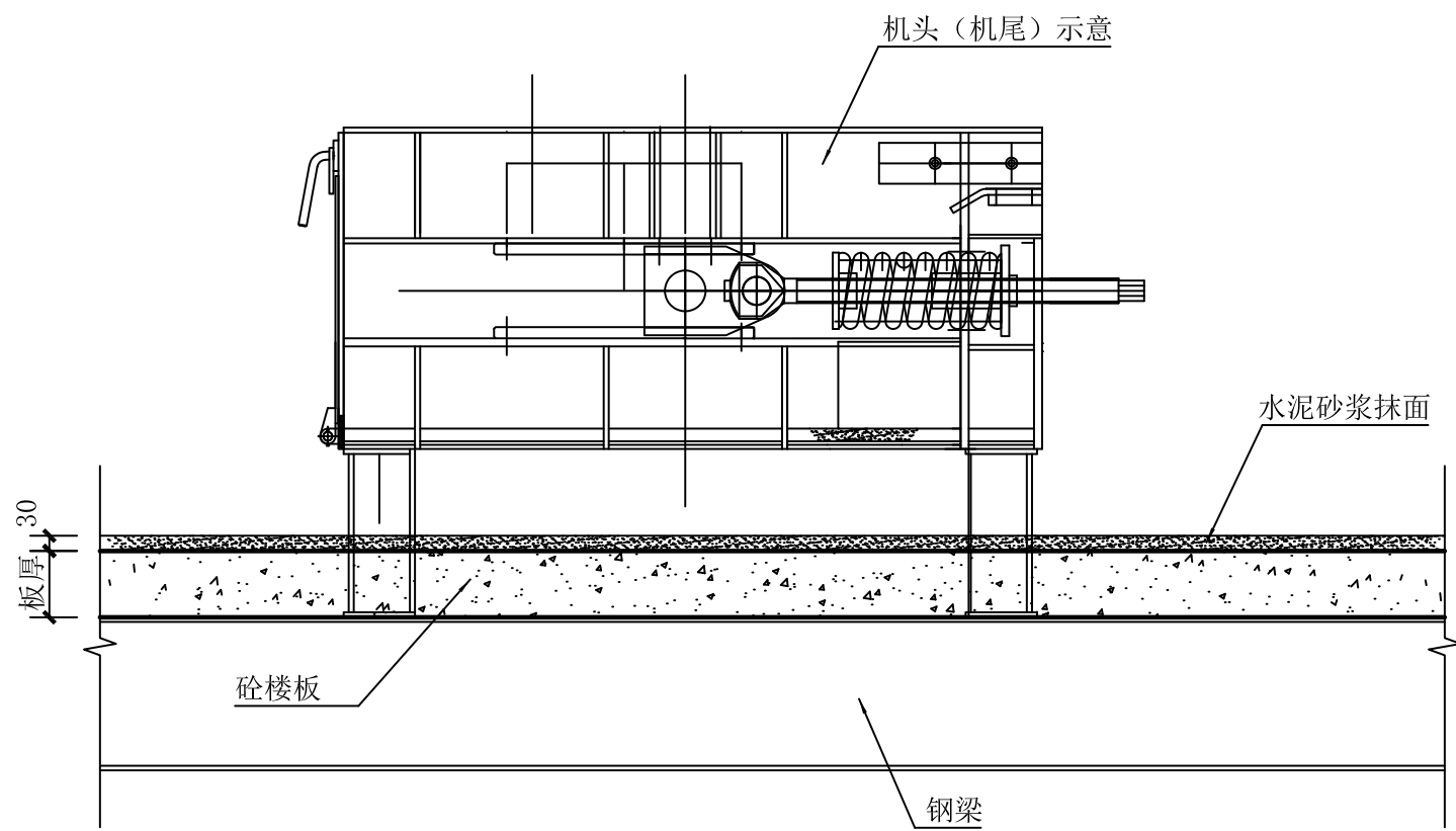
14 刮板、皮带机头机尾（支腿式）处楼板细部做法示意图
