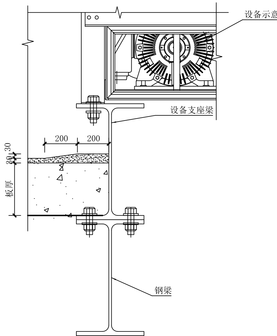
离心机、破碎机支座处楼板细部做法示意图
