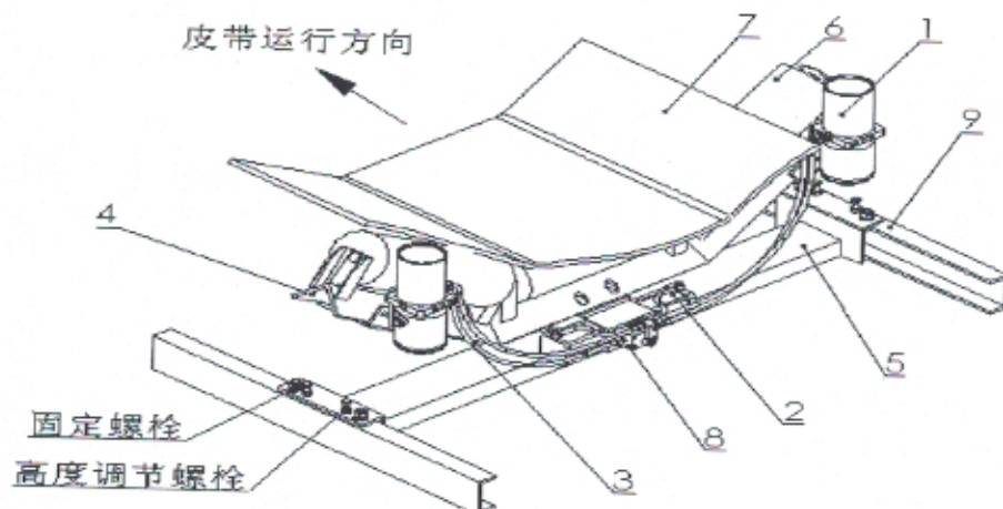
集成上液压调正器安装示意图
